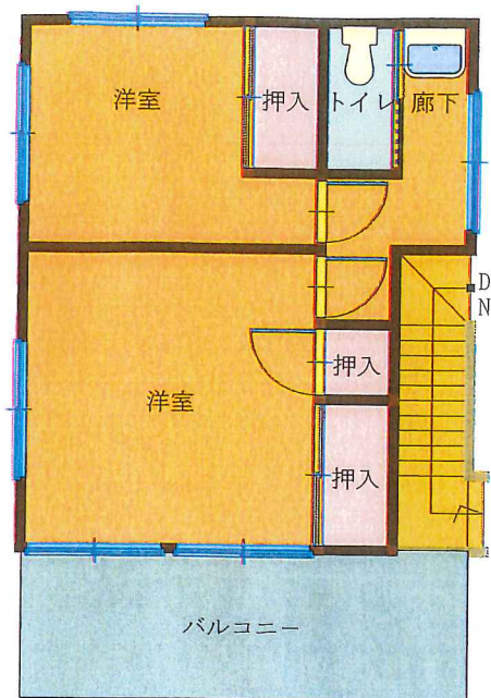
2F 平面図
