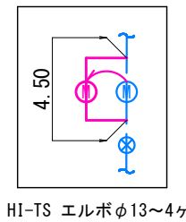
メーター移設 I (⑤横森宅) Co舗装
