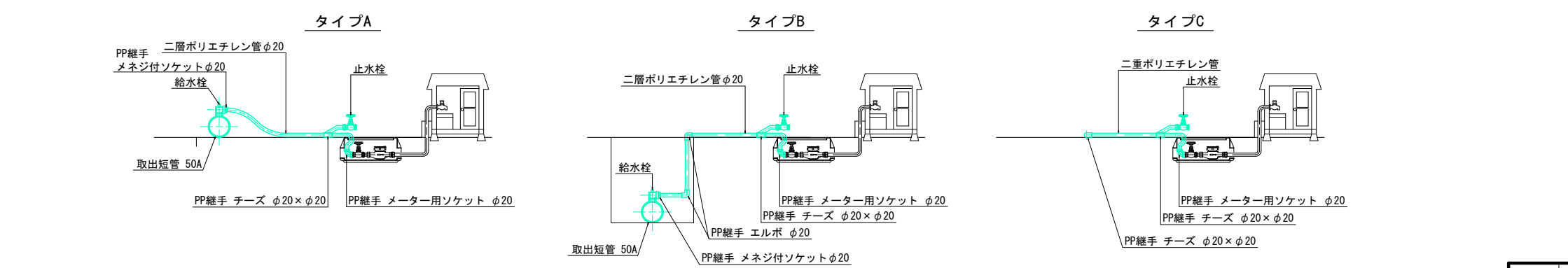
仮設給水切替標準図 S-Free
