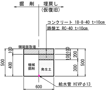
宅内Co舗装道 (メーター移設時)
