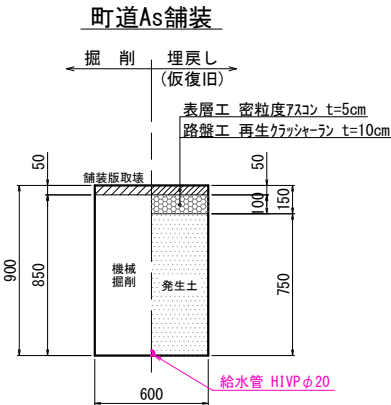
給水管土工定規図 S=1/20
