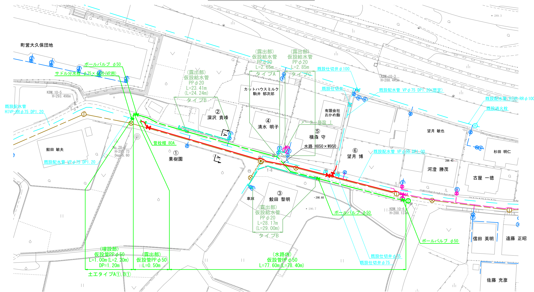
仮設管平面図 S=1/300
