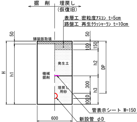
町道As舗装道
