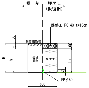
土エタイプA 町道As舗装道 (仮設置時)
