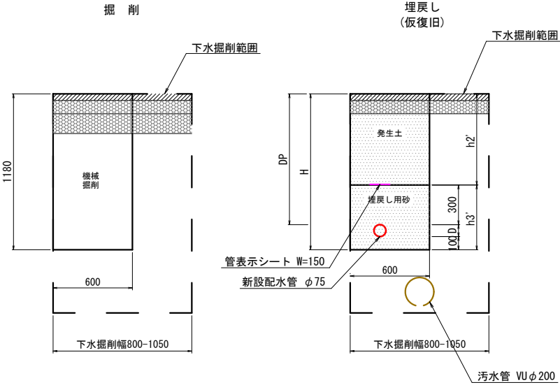
町道下水掘削幅内
