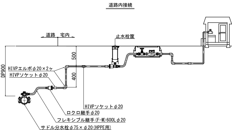
給水管取出し標準図 S=Free
