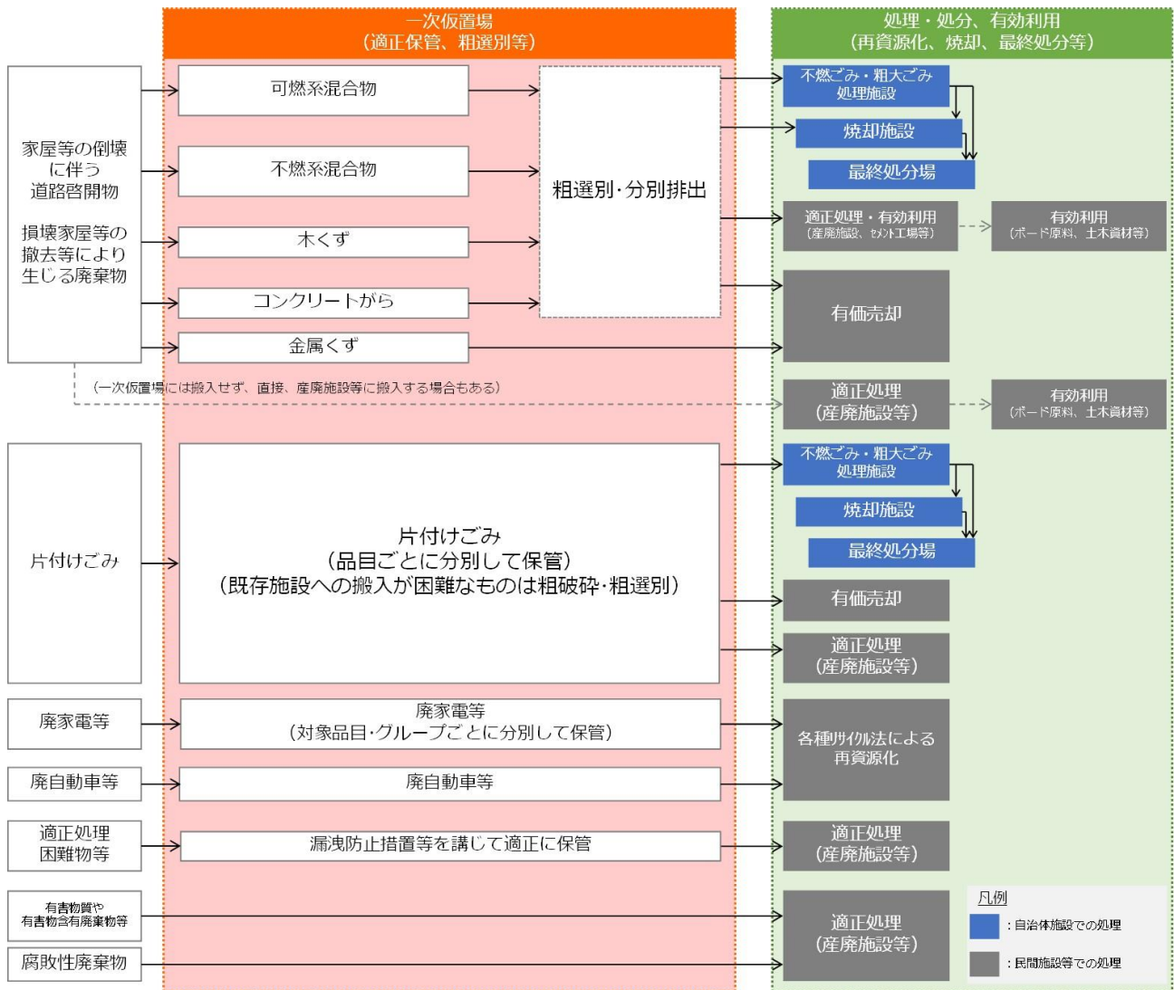
図表 6-15 災害廃棄物の処理フロー
