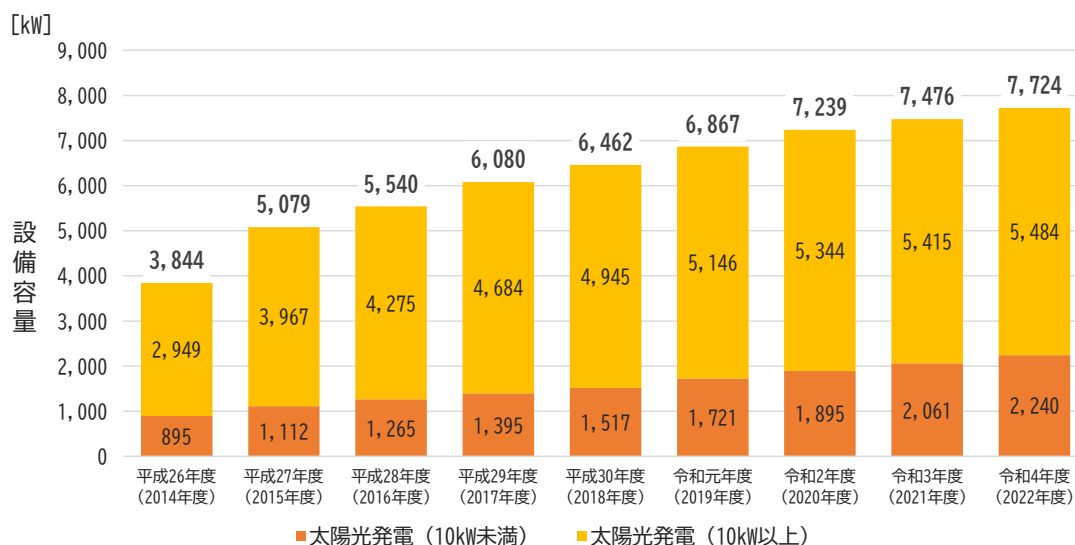
図 25 再生可能エネルギーの導入設備容量の推移（累積）
