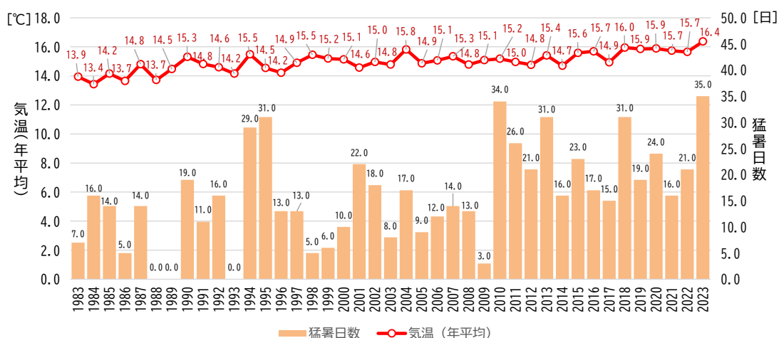
図 10 気温 (年平均) および猛暑日の推移
